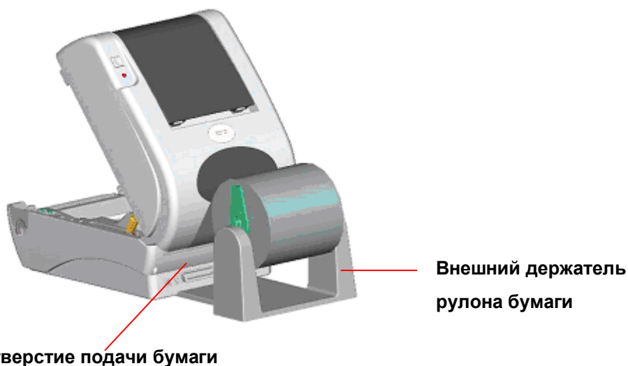
Рис. 10. Установка внешнего держателя рулона этикеток (I)
